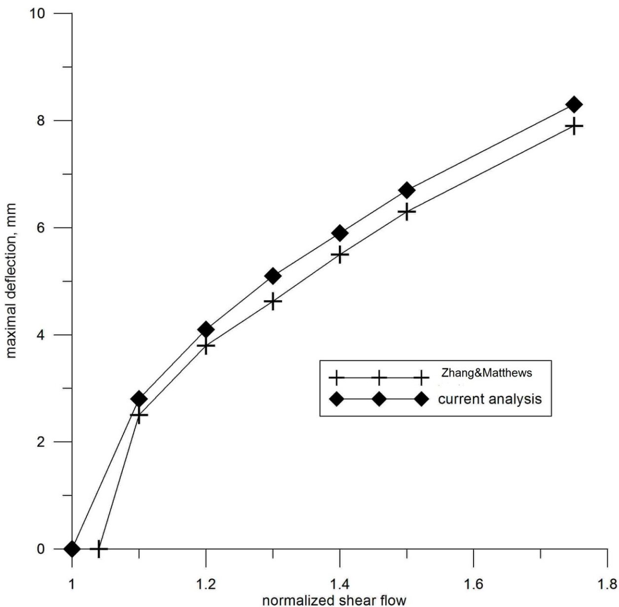
Рис. 6.3. Максимальный прогиб в центре пластины.
