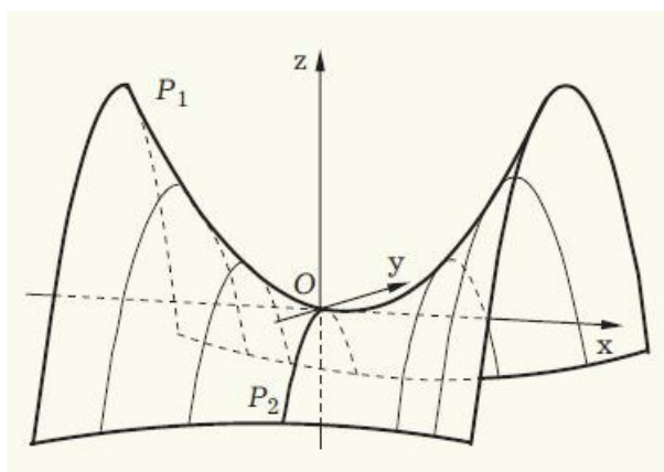
Рис. 5.23. Гиперболический параболоид.
