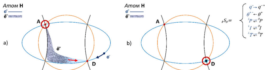
Рис. 11 (а и б). Концепция движения фундаментально-сцепленных фермионов в самосогласованном частице-солитонном атоме водорода протии. На рисунке 11а слева изображены: как электрон (частицы) двигающийся, по часовой стрелке, по траектории отличной от окружности и стремящейся к эллиптической в {}^LST и позитрон ( t -солитон) двигающийся, против часовой стрелки (по s -орбитали), по гиперболическим t -солитонным траекториям в {}^DST - приближаются к точке локализации – D ( tS_D = \pm \frac{1}{2} ) в {}^AST . На рисунке 11б справа показан момент максимального сближения проекций электрона (частицы) и позитрона (частицы) в правой нижней точке локализации – D ( tS_D = \pm \frac{1}{2} ) в {}^AST , когда между электроном частицей и позитроном частицей - становится возможным идеальное обменное взаимодействие.
