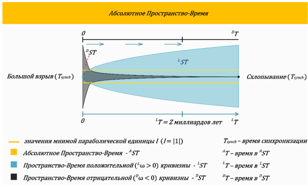
Рис. 1. Трех пространственно-временная модель строения Вселенной. В обобщенном Паракомплексном Абсолютном пространстве-времени {}^4ST в момент Большого Взрыва ( BB ) синхронно (в T_{synch} ) рождаются два взаимопрозрачных самосогласованных некоммутативных пространства-времени: постоянной положительной кривизны {}^LST и постоянной отрицательной кривизны {}^DST . В любой момент времени синхронизации T_{synch} произведение кривизны {}^L\omega пространства-времени {}^LST на кривизну {}^D\omega пространства-времени {}^DST равна мнимой параболической единице I [ {}^L\omega(T_{synch}) \cdot {}^D\omega(T_{synch}) = I ], где I = |1| . Судьба обоих пространств-времен {}^LST и {}^DST - предрешена, они исчезнут также синхронно (в T_{synch} ), в момент Схлопывания ( Cr ).
