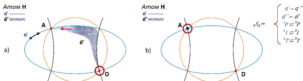
Рис. 12 (а и б). Концепция движения фундаментально-сцепленных фермионов в самосогласованном частице-солитонном атоме водорода протии. На рисунке 12а слева изображены: как электрон (частицы) двигающийся, по часовой стрелке, по траектории отличной от окружности и стремящейся к эллиптической в {}^LST и позитрон ( t -солитон) двигающийся, против часовой стрелки (по s -орбитали), по гиперболическим t -солитонным траекториям в {}^DST - приближаются к точке локализации – A ( tS_A = \pm \frac{1}{2} ) в {}^AST . На рисунке 12б справа показан момент максимального сближения проекций электрона (частицы) и позитрона (частицы) в левой верхней точке локализации – A ( tS_A = \pm \frac{1}{2} ) в {}^AST , когда между электроном частицей и позитроном частицей - становится возможным идеальное обменное взаимодействие.
