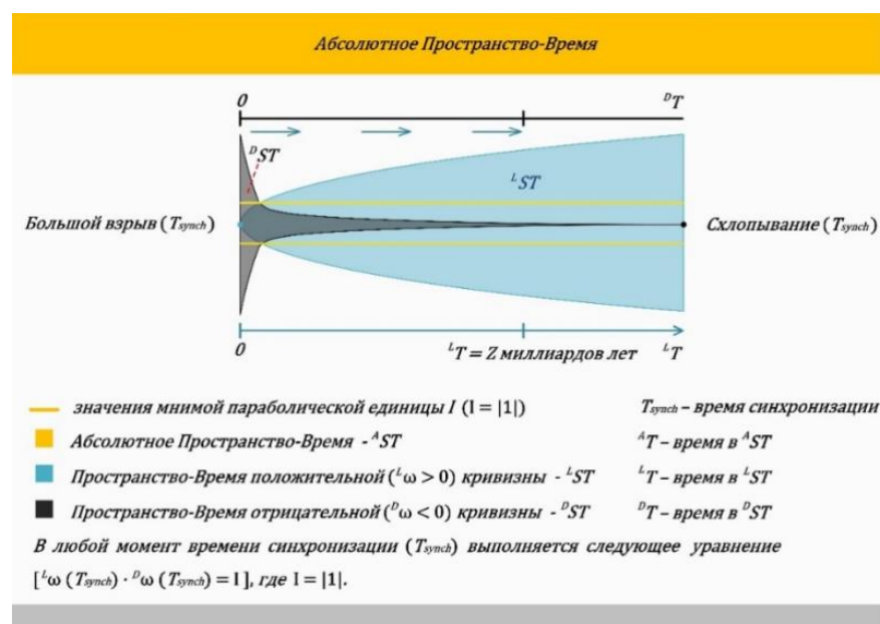
Графический абстракт: трех пространственно-временная модель строения Вселенной.
