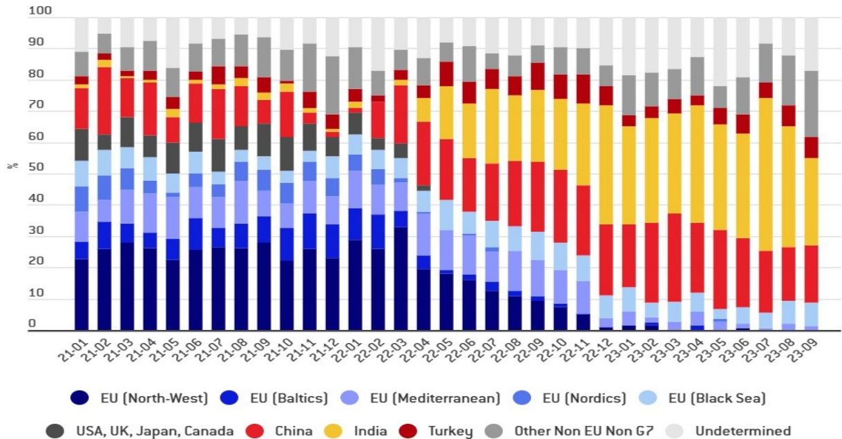
Ежемесячный экспорт российской нефти по стране прибытия. Источник: Bloomberg, CREA, Bruegel computations
