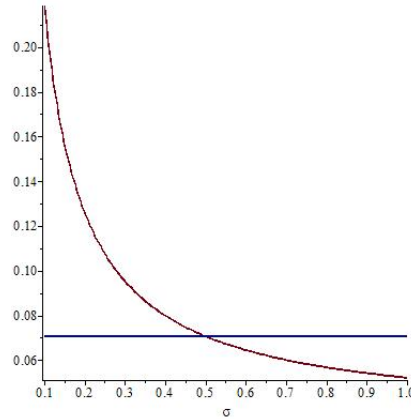
Рис. 5: Пересечение графиков v_1 и v_2
