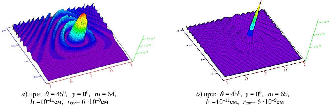
Рис. 27. Объемные диаграммы упругого рассеяния электронов на многослойной поверхности монокристалла, рассчитанные по формуле (155) при различных значениях параметров \vartheta , l_1 , n_1 и r_{\text{cor}}
