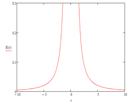
Рис. 10. График функции (59) E_{vr}^{(+ab)}
