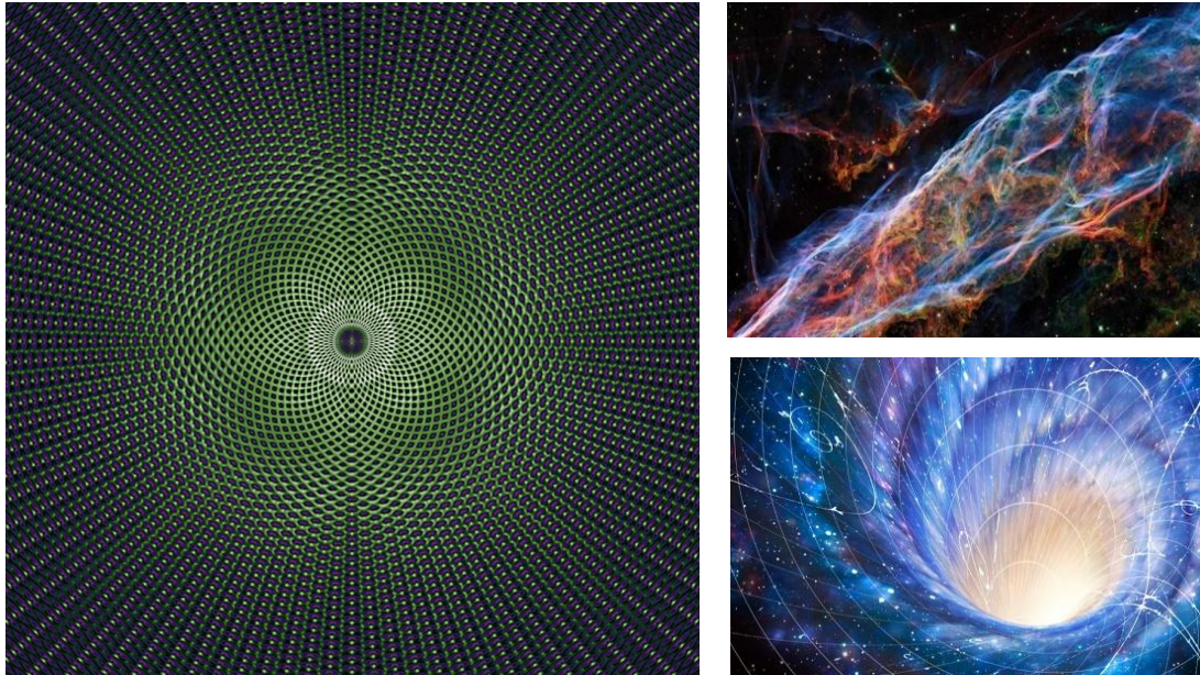
Рис. 8. Иллюстрация переплетения субконтных токов и противотоков в окрестности ядра свободного валентного «электрона»
