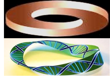
Рис. 33. Четырехсторонняя лента Мёбиуса и циркуляция свернутых в спираль субконт-антисубконтных токов по одной из ее сторон
