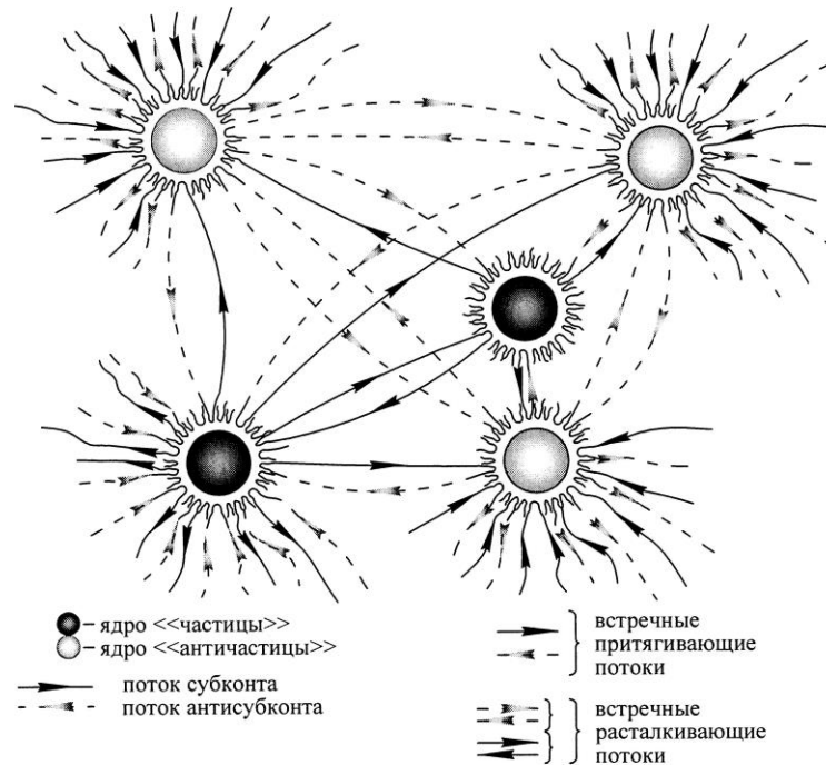
Рис. 31. Субконт - антисубконтные токи между ракиями «частиц» и «античастиц»
