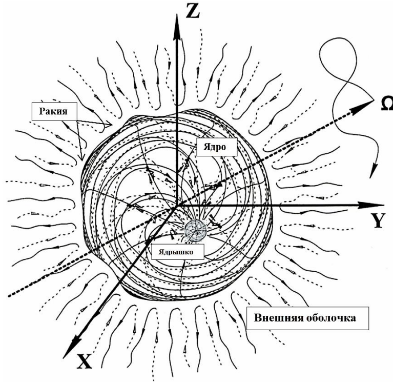
Рис. 1. Иллюстрация полностью геометризованной модели стабильного сферического вакуумного образования (в частности, свободного «электрона») с четырьмя явно выраженными областями:
