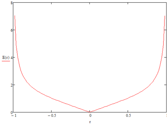
Рис. 16. График функции (80а) ускорения субконта (при условно принятых r_6 = 1 , c = 1 ) в случае, если внутри ядра «электрона» отсутствует внутреннее ядрышко
