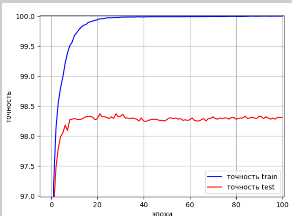
Рисунок 7. Эксперимент 2 (MNIST). Обучение 100 эпох.
