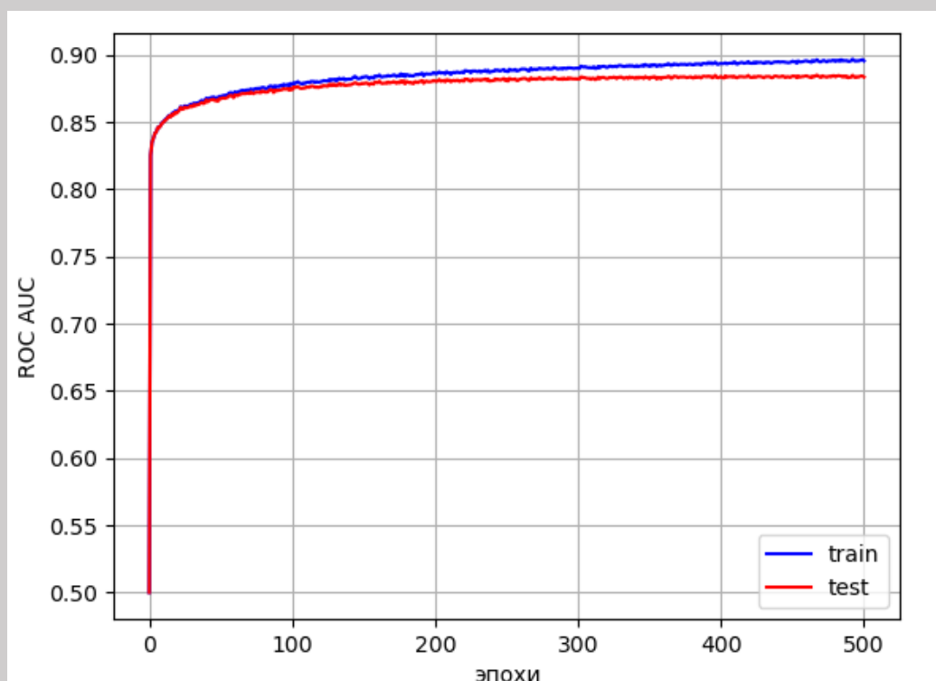
Рисунок 12. Тест 1. График обучения на датасете HIGGS.
