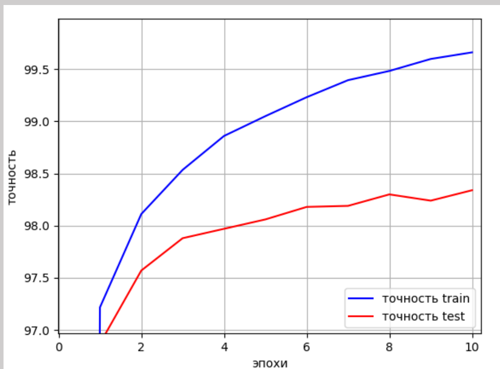
Рисунок 6. Эксперимент 2 (MNIST). Обучение 10 эпох.
