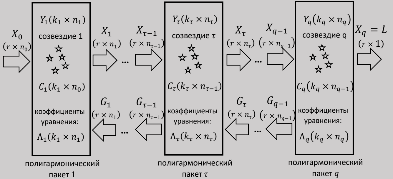
Рисунок 1. Полигармонический каскад
