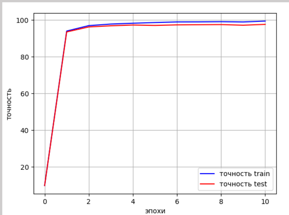
Рисунок 10. Эксперимент 4 (MNIST). Обучение каскада из 500 слоёв. Посмотрим более детально на показатели точности на графике.
