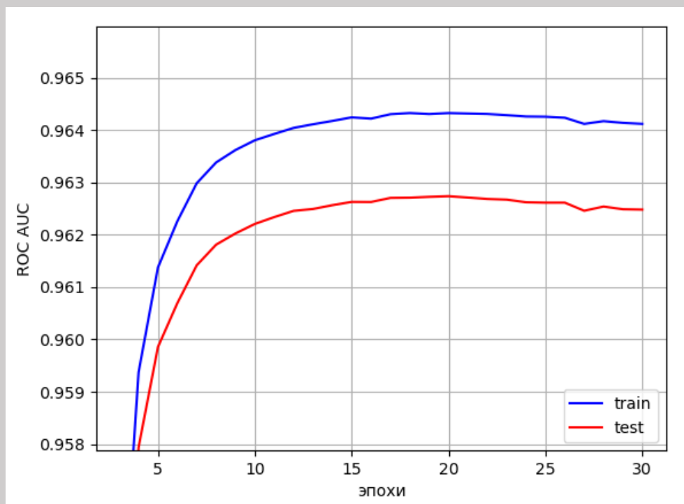
Рисунок 18. Тест 2. Обучение на датасете Epsilon.
