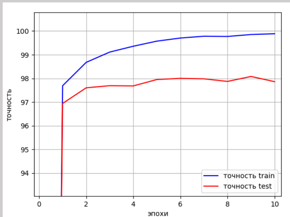
Рисунок 9. Эксперимент 3 (MNIST). Обучение каскада из 100 слоёв.
