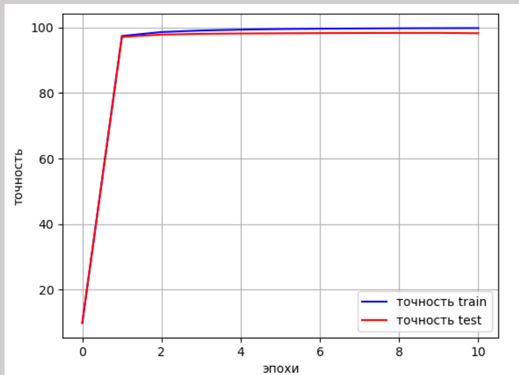
Рисунок 4. Эксперимент 1. График обучения на датасете MNIST.
