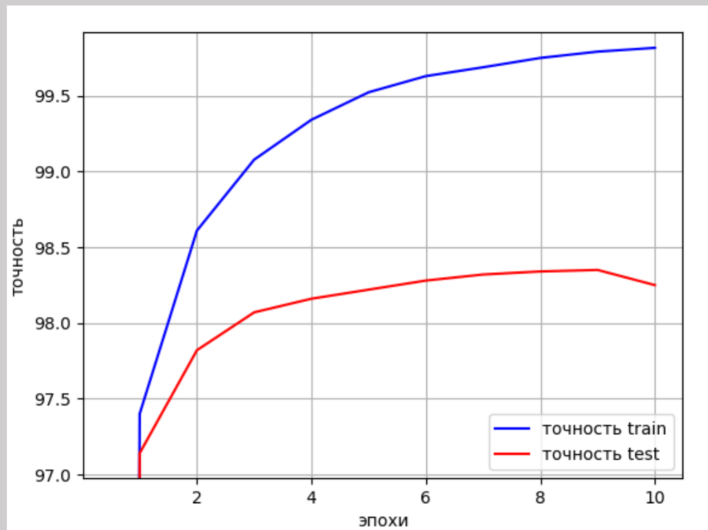
Рисунок 5. Эксперимент 1. График обучения на датасете MNIST (в масштабе).
