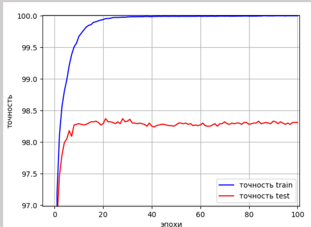
Рисунок 7. Эксперимент 2 (MNIST). Обучение 100 эпох.
