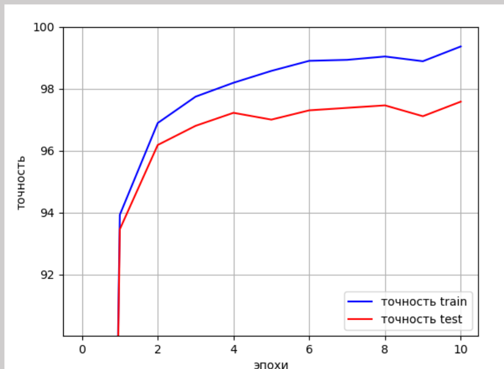
Рисунок 11. Эксперимент 4 (MNIST). Обучение каскада из 500 слоёв (график в масштабе).
