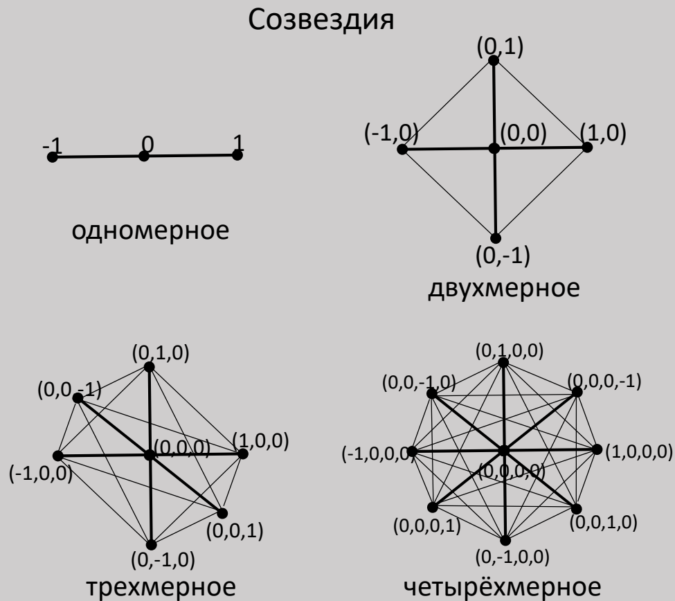
Рисунок 2. Принципы формирования созвездий на основе гипероктаэдров.
