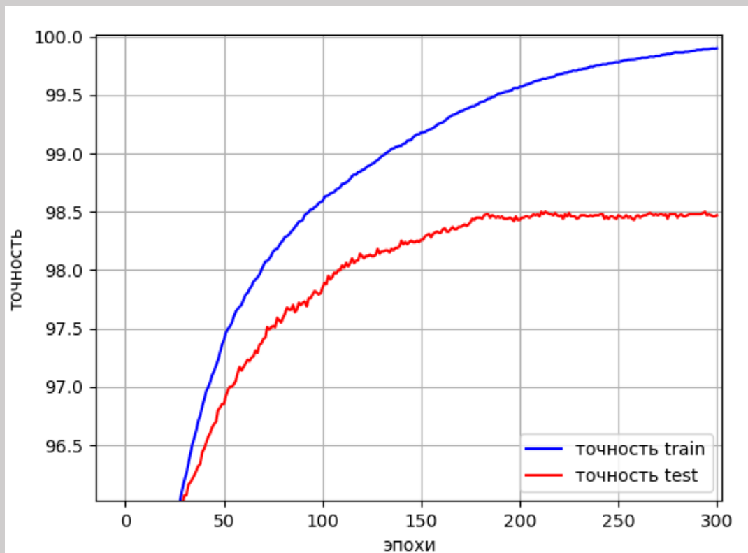
Рисунок 8. Эксперимент 2 (MNIST). Специально замедленное обучение.
