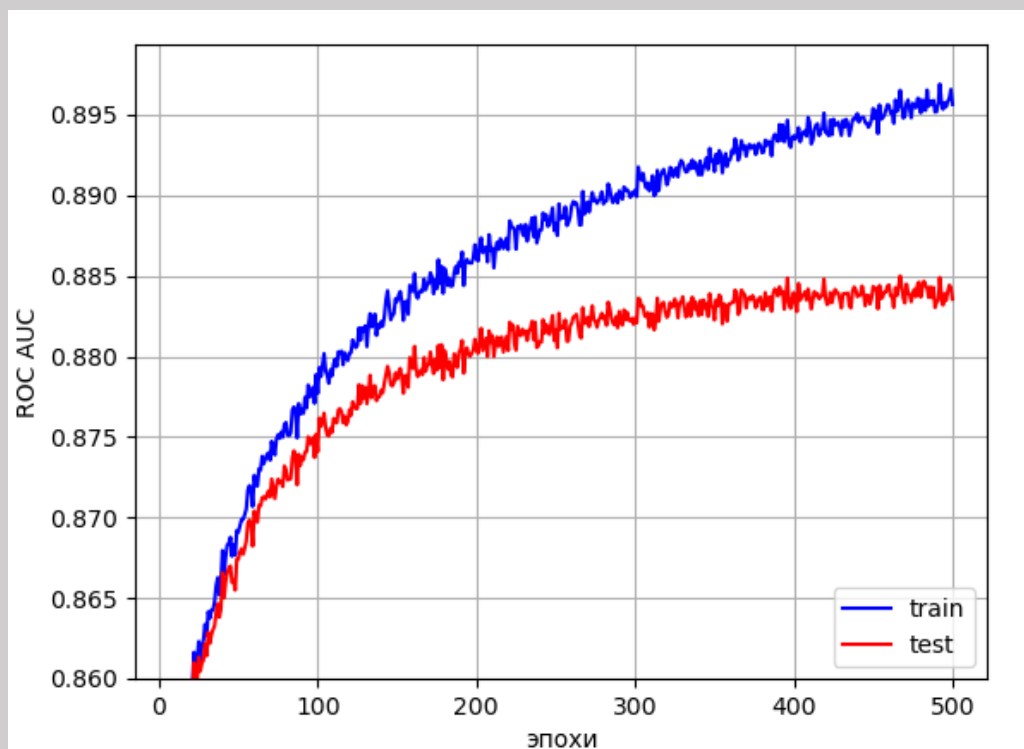
Рисунок 13. Тест 1. График обучения на датасете HIGGS (в масштабе).
