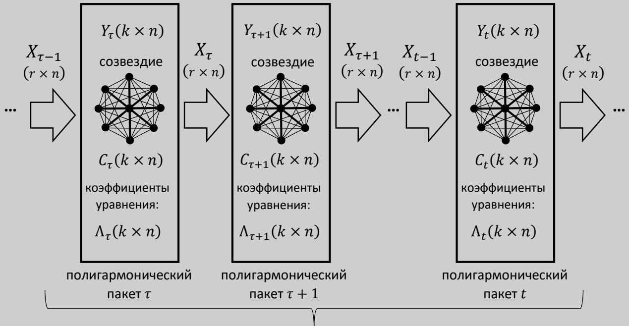
Рисунок 3. Фрагмент полигармонического каскада
