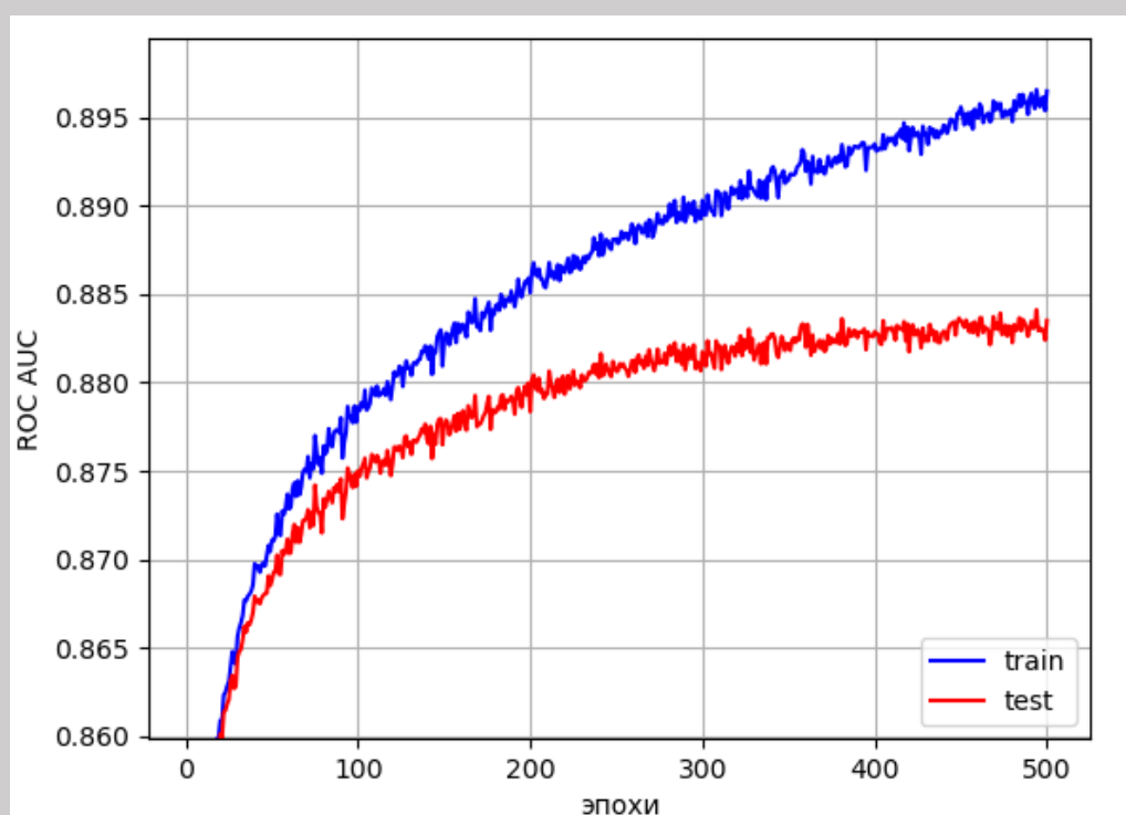
Рисунок 15. Тест 2. График обучения на датасете HIGGS (в масштабе).
