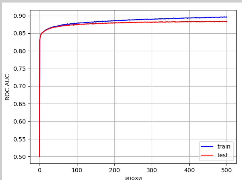
Рисунок 14. Тест 2. График обучения на датасете HIGGS.
