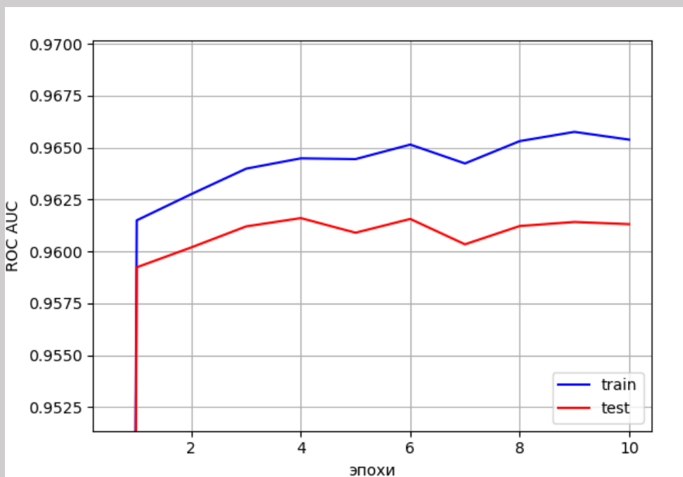
Рисунок 17. Тест 1. Обучение на датасете Epsilon (в масштабе).
