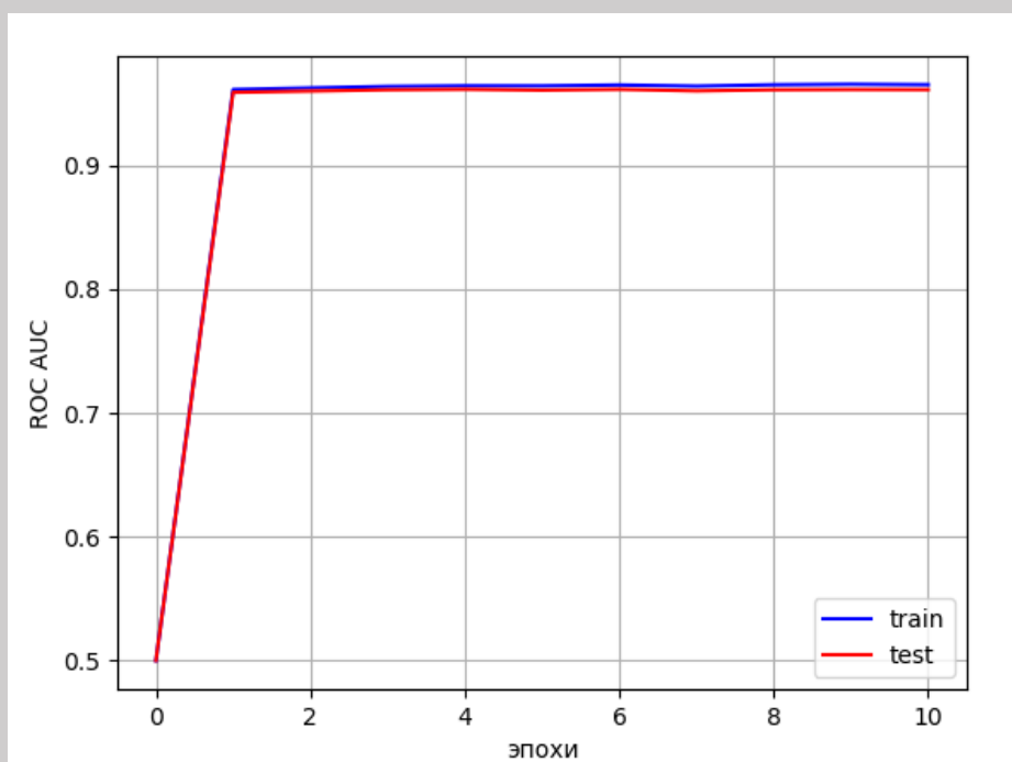
Рисунок 16. Тест 1. Обучение на датасете Epsilon.
