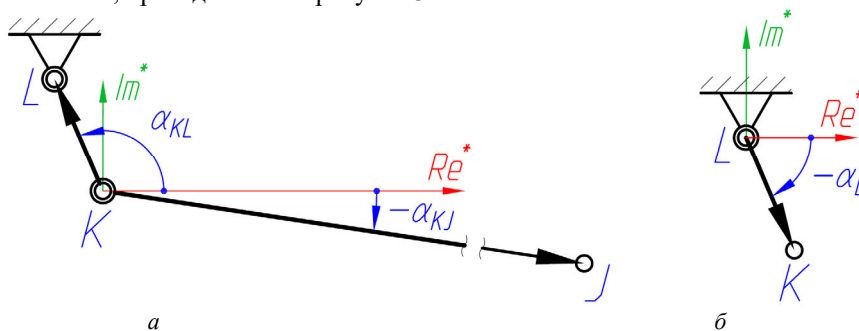
Рисунок 3. – Расчетные схемы к оценке угла закручивания сайлентблоков в шарнирах
