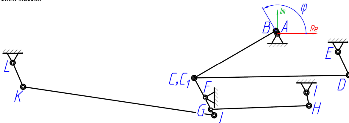
Рисунок 2. – Кинематическая схема механизма привода очистки зерноуборочного комбайна
