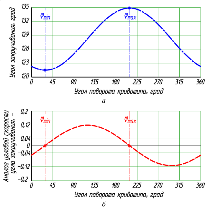
a – угол закручивания; b – аналог угловой скорости угла закручивания Рисунок 4. – График изменения угловых параметров для сайлентблока в шарнире K механизма
