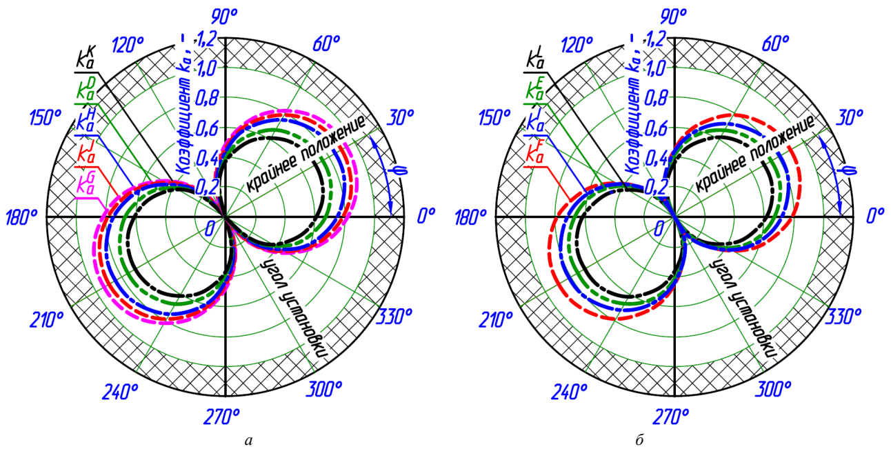
a – результаты расчета в шарнирах звеньев; б – результаты расчета в шарнирах опор Рисунок 5. – Годографы изменения коэффициента угла закручивания сайлентблоков в шарнирах механизма привода очистки
