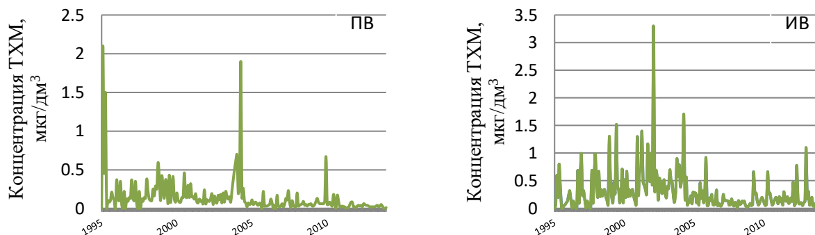
Рисунок 1 - Временные ряды содержание ТХМ в створах водоисточника (реки) поверхностного (ПВ) и инфильтрационного водозаборов (ИВ)
