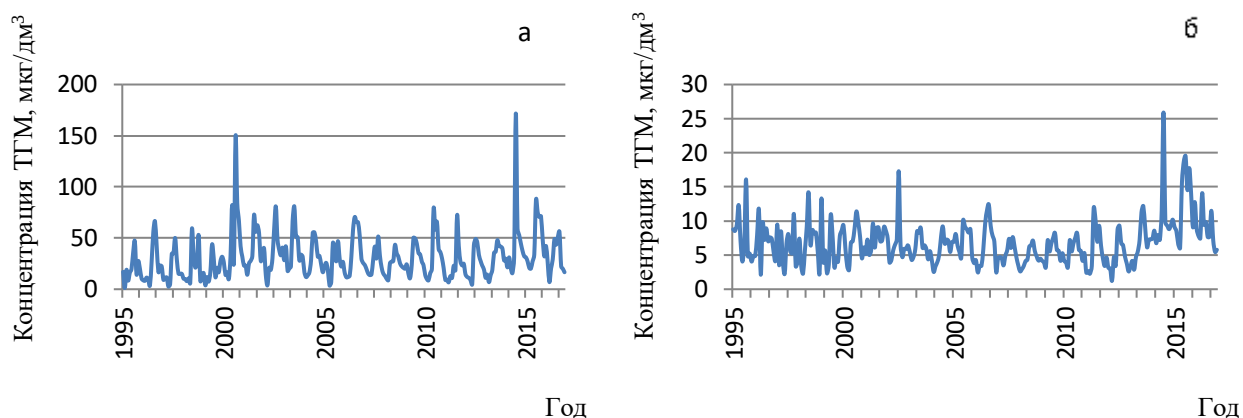
Рисунок 2 – Временные ряды суммарного содержания ТГМ в РЧВ водозаборов ПВ (а) и ИВ (б) (1995 - 2016 гг.)
