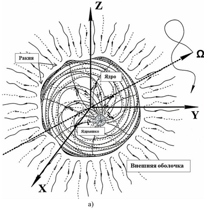
Рис. 1: (повтор рис. 1 в [7]) Иллюстрация стохастической метрико-динамической модели стабильного сферического вакуумного образования («корпускулы» в частности, «электрона»), в окрестности его ядра с четырьмя явно выраженными областями:
