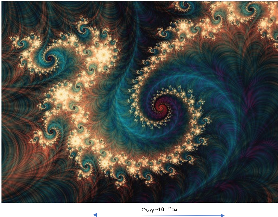
Рис. 11: Фрактальная иллюстрация того, как внешняя оболочка e_j^+ -«прото-кварка» окружает его мизерное ядрышко (яЭПК) с предполагаемым радиусом r_7 \sim 10^{-24} см, и как циклон увлекается за его хаотическим перемещением. Вместе с тем ближняя к ядрышку часть внешней оболочки отчасти входит в эффективный размер самого яЭПК r_{7eff} \sim 10^{-17} см (смотрите рис. 7) и влияет на величину основных характеристик исследуемого случайного процесса 2\sigma_r^2/\tau_{rcor}
