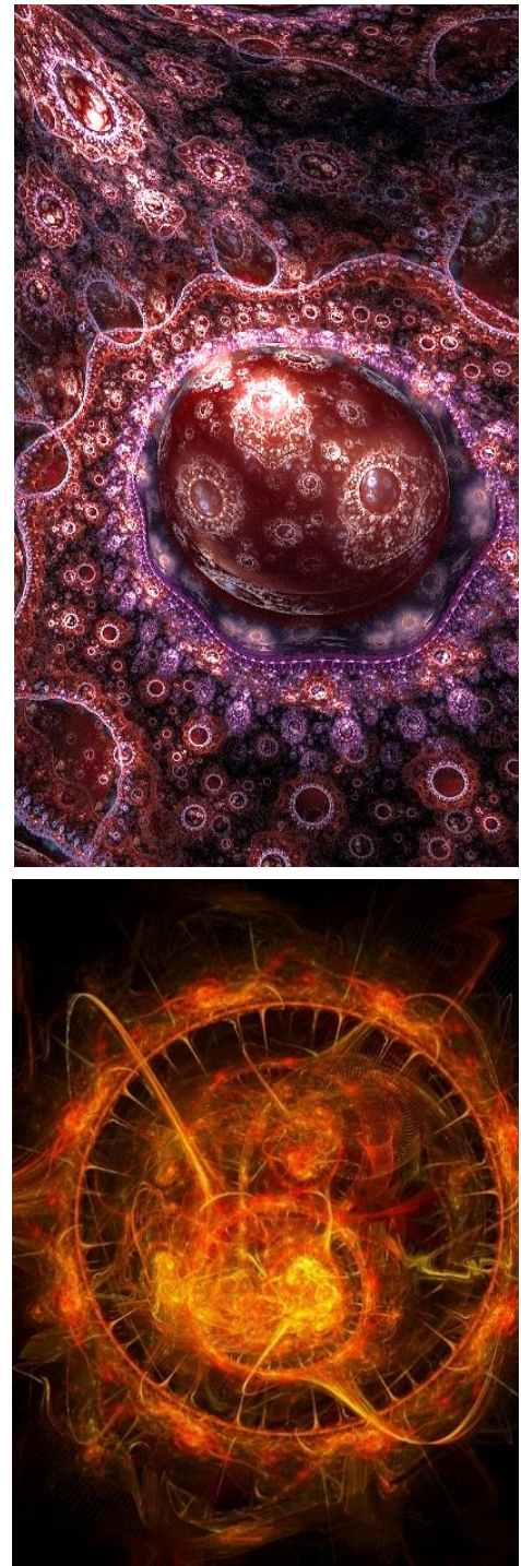
Рис. 12: Фрактальные иллюстрации бурлящего ядра «атома водорода» и размытой внешней оболочки хаотически блуждающего ядрышка e_j^+ -«прото-кварка»
