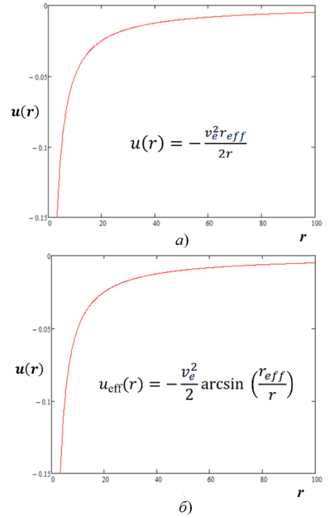
Рис. 10: а) График функции u(r) (211) при условно принятых v_e = r_{eff}=1 ; б) График функции u(r) (221) при условно принятых v_e = r_{eff}=1
