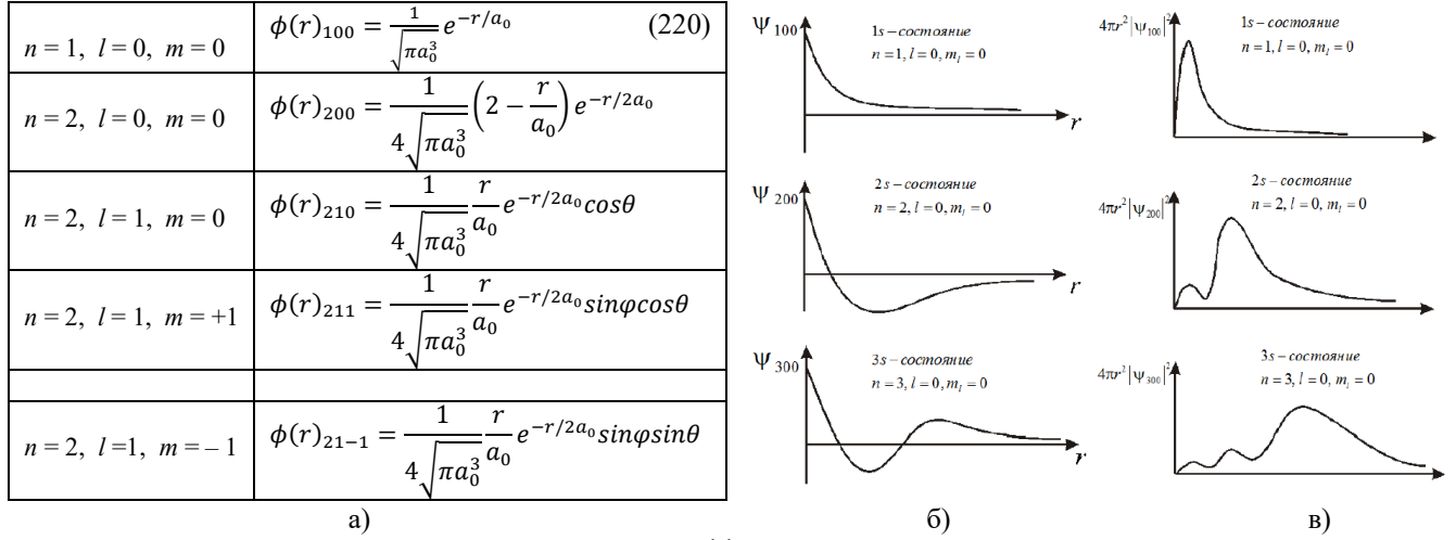
Рис. 9: а) Волновые функции яЭПК в «атоме водорода» \phi(r)_{n,l,m} при подстановке различных значений квантовых чисел n, l, m в выражение(217); б) Графики трех волновых функций \phi(r)_{n,l,m} = \psi(r)_{nlm} (217); в) Плотности распределения вероятности 4\pi r^2 |\phi(r)_{n,l,m}|^2 того, что яЭПК находится в сферическом слое 4\pi r^2 dr
