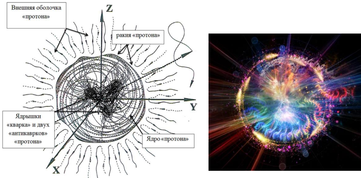
Рис. 2: Визуализированная стохастическая метрико-динамическая модель в среднем вогнутого сферического стабильного вакуумного образования (в частности, p_i^- -«протона»), состоящего из 2-х цветных «антикварков» и одного «кварка» (40) – (48). Внутренние ядрышки (т.е., цветные «прото-кварки» и «прото-антикварки» этих вакуумных образований находятся в постоянном хаотическом перемещении относительно друг друга и относительно общего центра ядра p_i^- -«протона»
