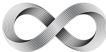
Рисунок 1 Лента Мёбиуса
