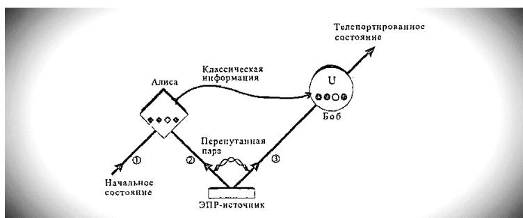
Рис. 1. Принцип квантовой телепортации мезо- и макроскопических состояний.
