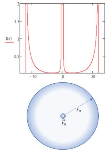
Рис. 1: График функции относительного удлинения l_r^{(+)}(24) , определяющей относительное удлинение вакуума в радиальном направлении
