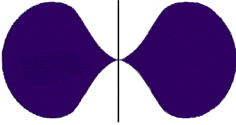
Рис.7. Черная Дыра Керра при угловом моменте J > \frac{\gamma M^2}{c} в разрезе вдоль плоскости, проходящей через ось вращения. Цветом обозначена область эргосферы.
